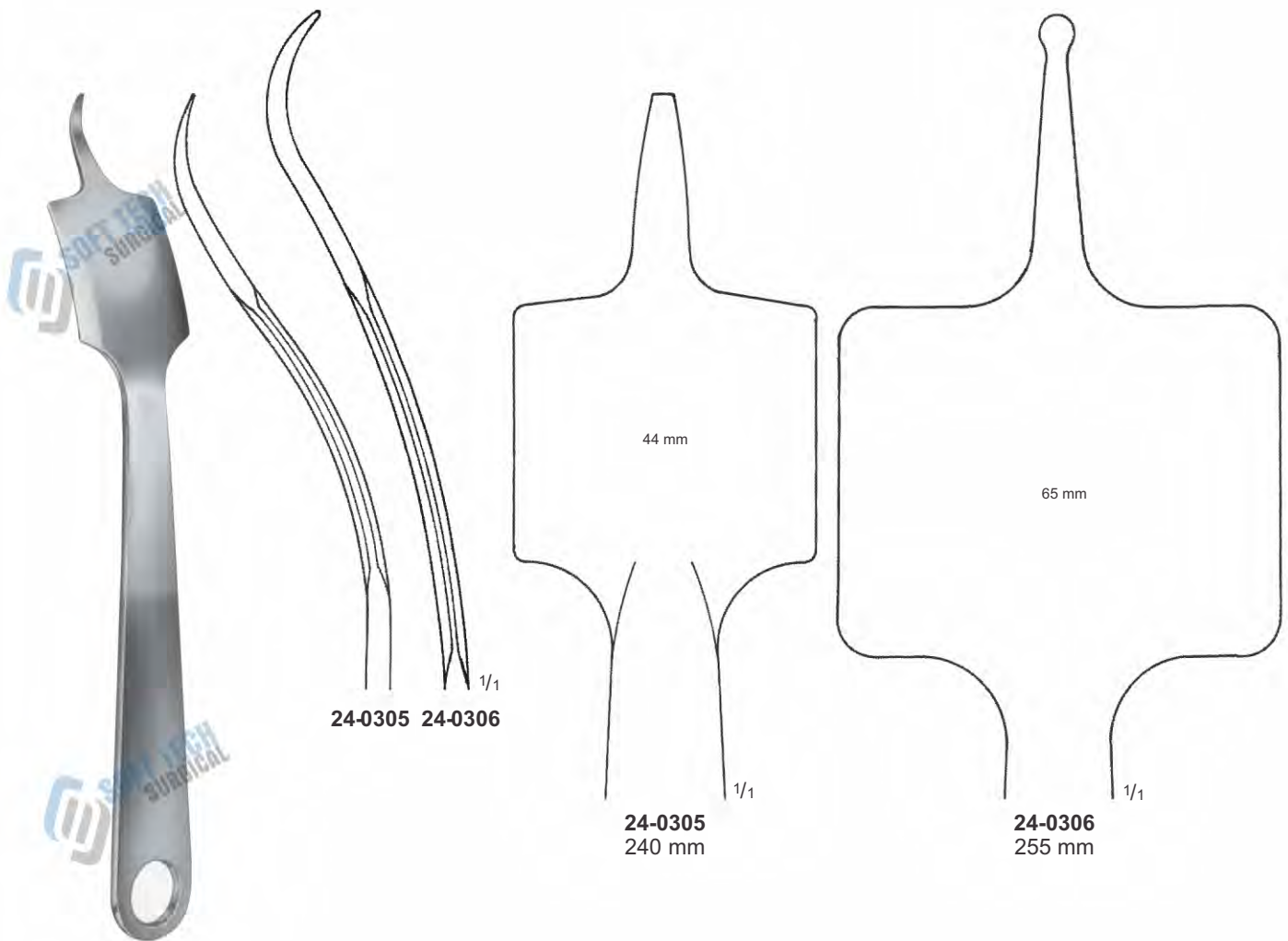
VERBRUGGE- MÜLLER BONE LEVER
