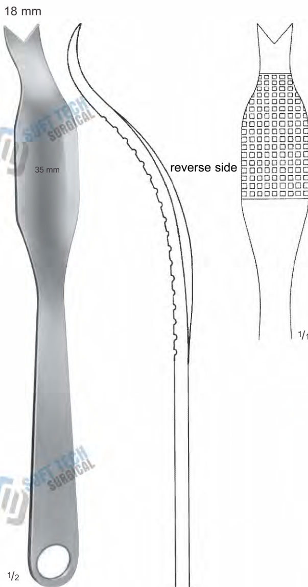
SCHUMACHER BONE LEVER 24-0350 290 mm
